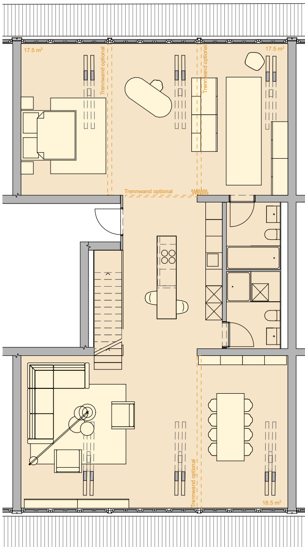
4.OG
